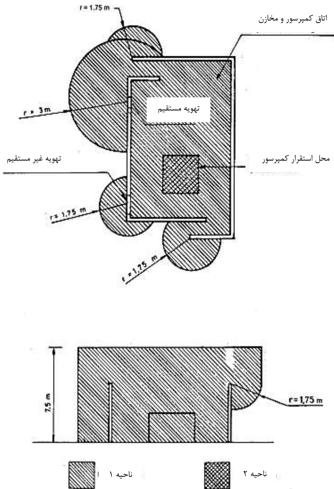
شکل ۹- کمپرسور و مخازن ذخیره در فضای بسته
